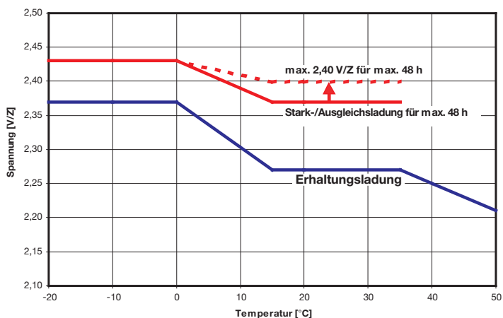
Bild 3: A 400/FT; Ladespannung über der Temperatur
