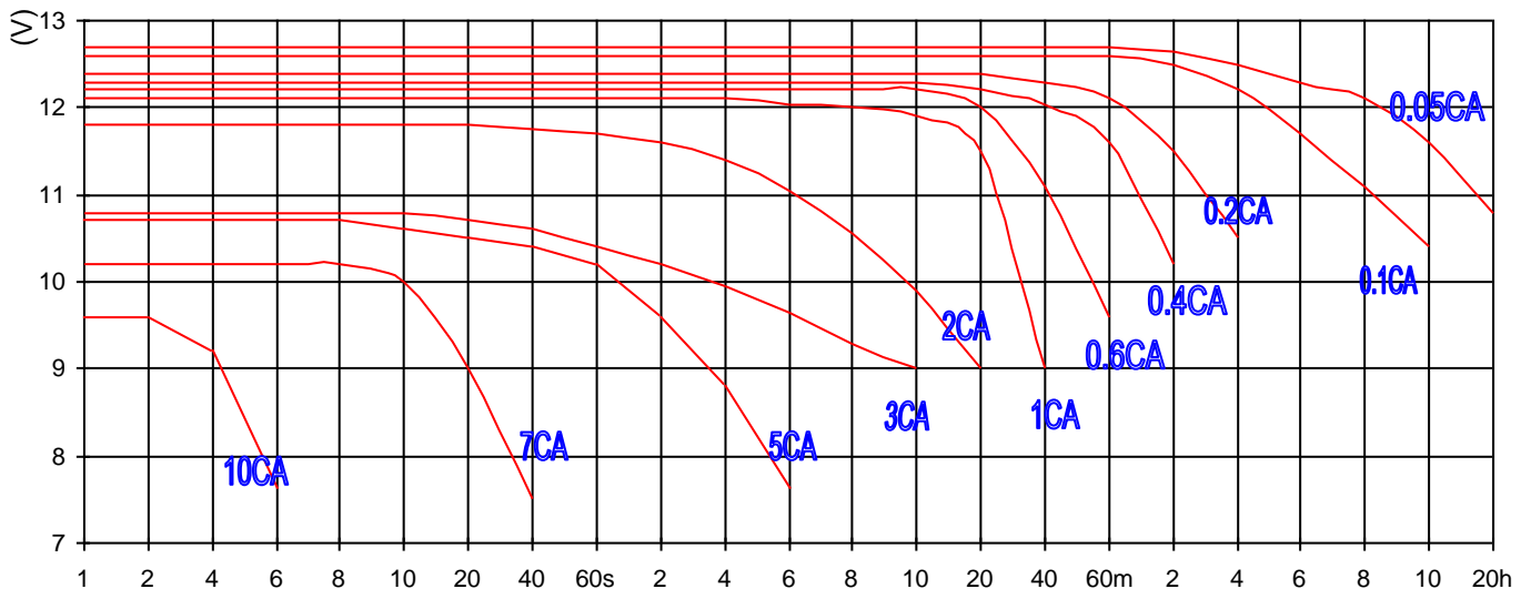
Abb.3:Entlade-Kennlinien (für C = 2,3 Ah)
