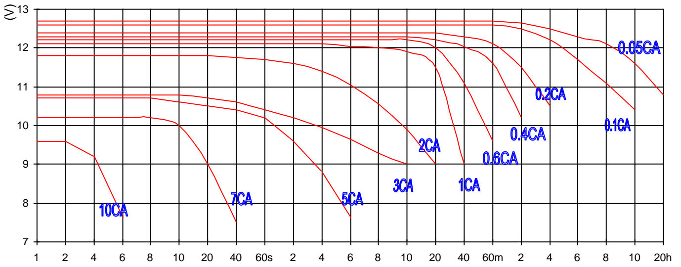
Abb.3: Entlade-Kennlinien (C=18)
